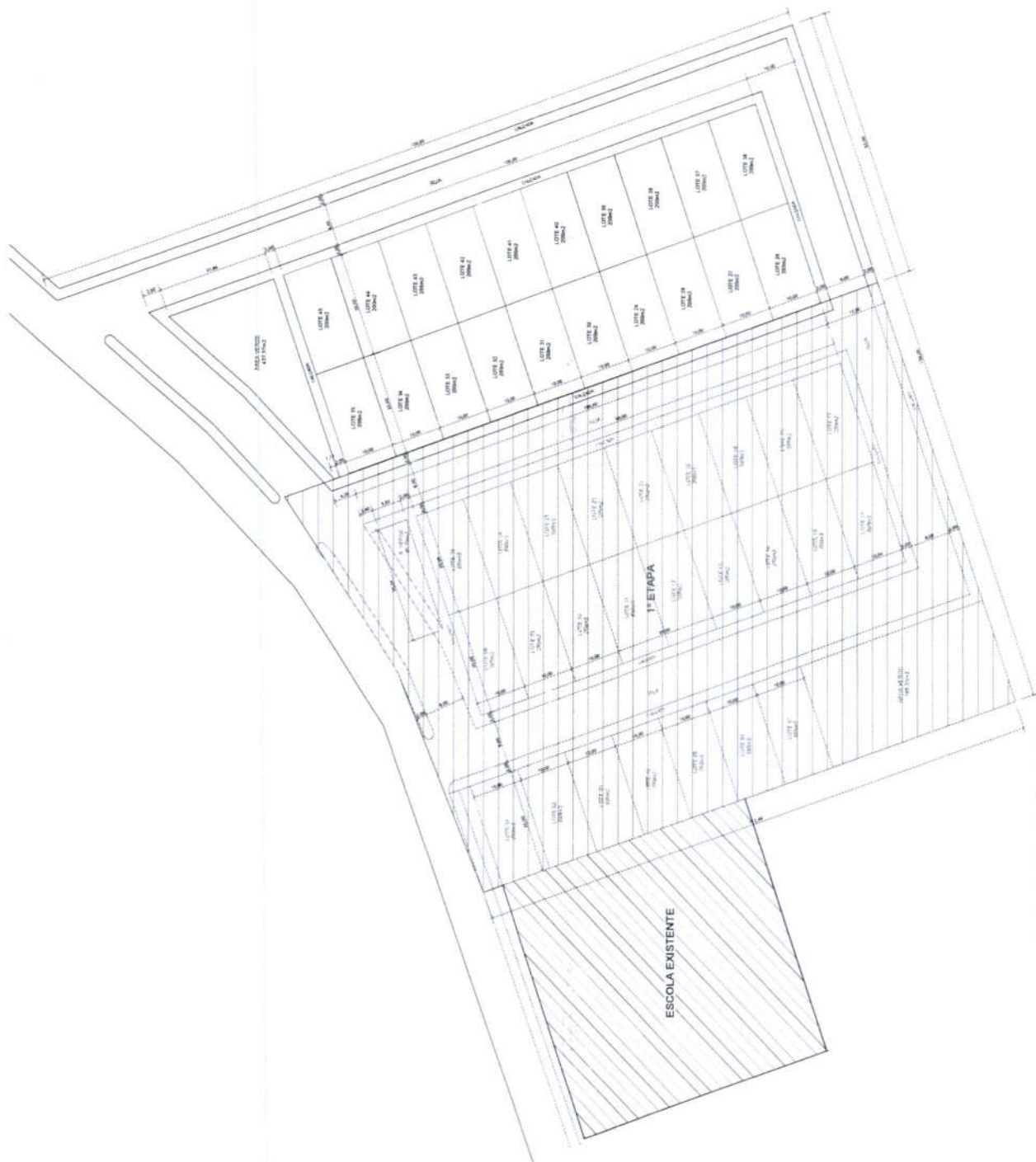
1 PLANTA DE IMPLANTAÇÃO - 2ª ETAPA ESCALA 1:500
