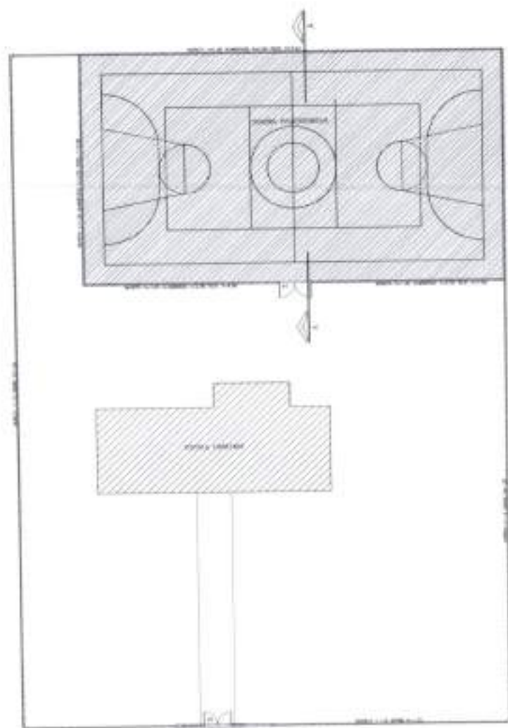
1 PLANTA BAIXA - CONSTRUÇÃO 1:500 1:50
