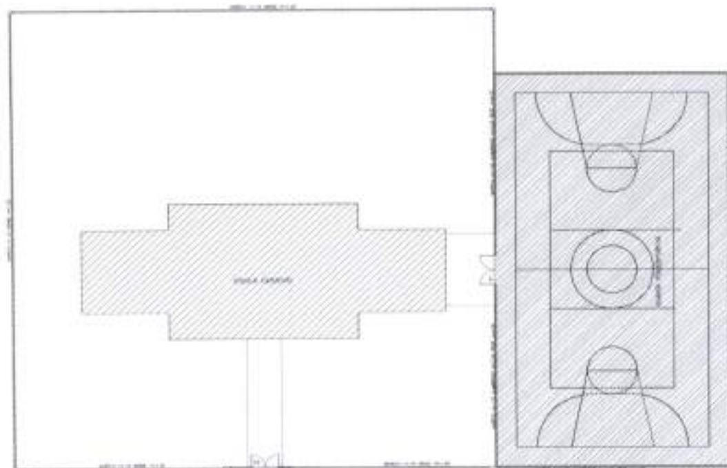
1 PLANTA BAIXA - CONSTRUÇÃO
