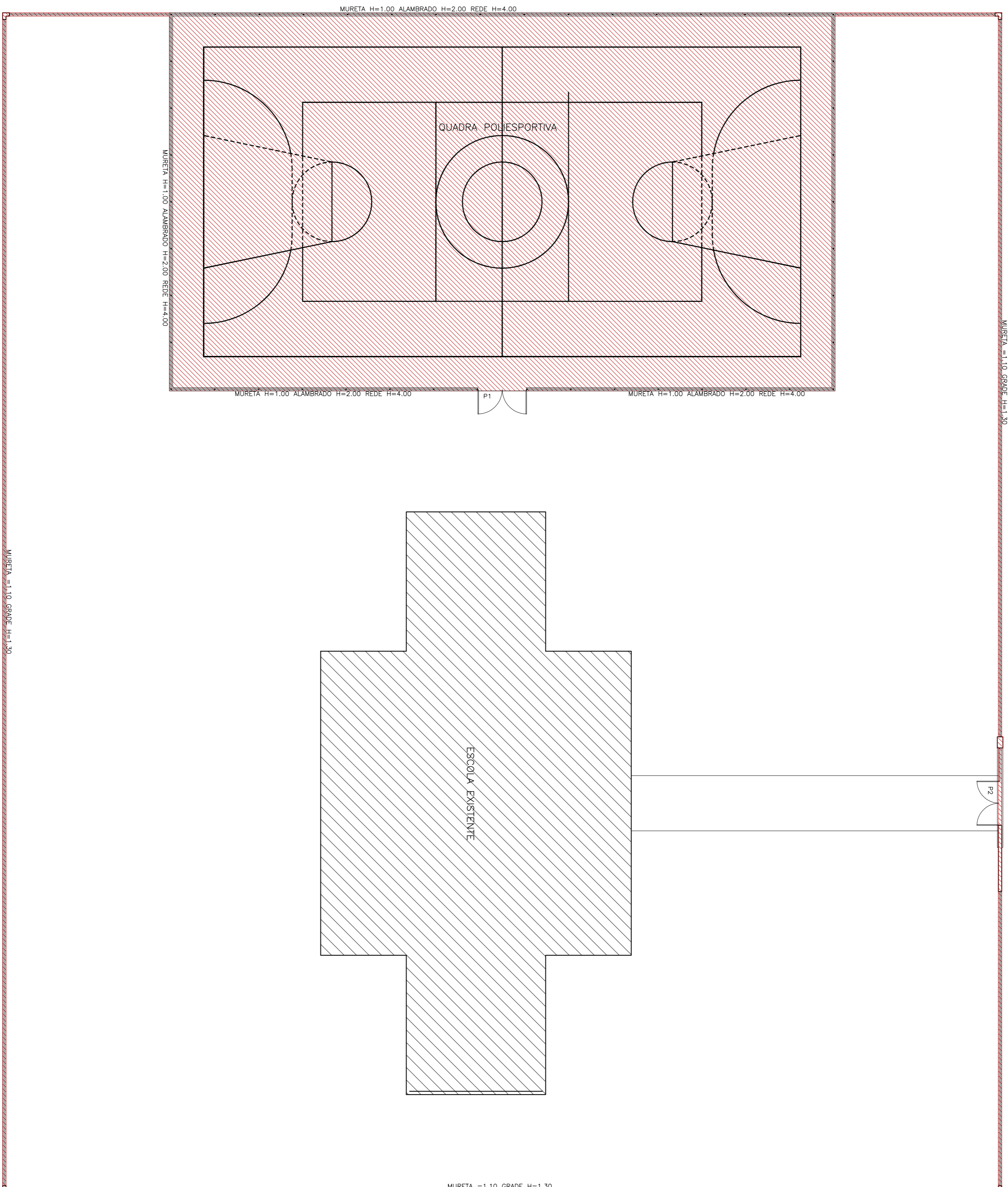
1 PLANTA BAIXA - CONSTRUÇÃO ESCALA 1:125
