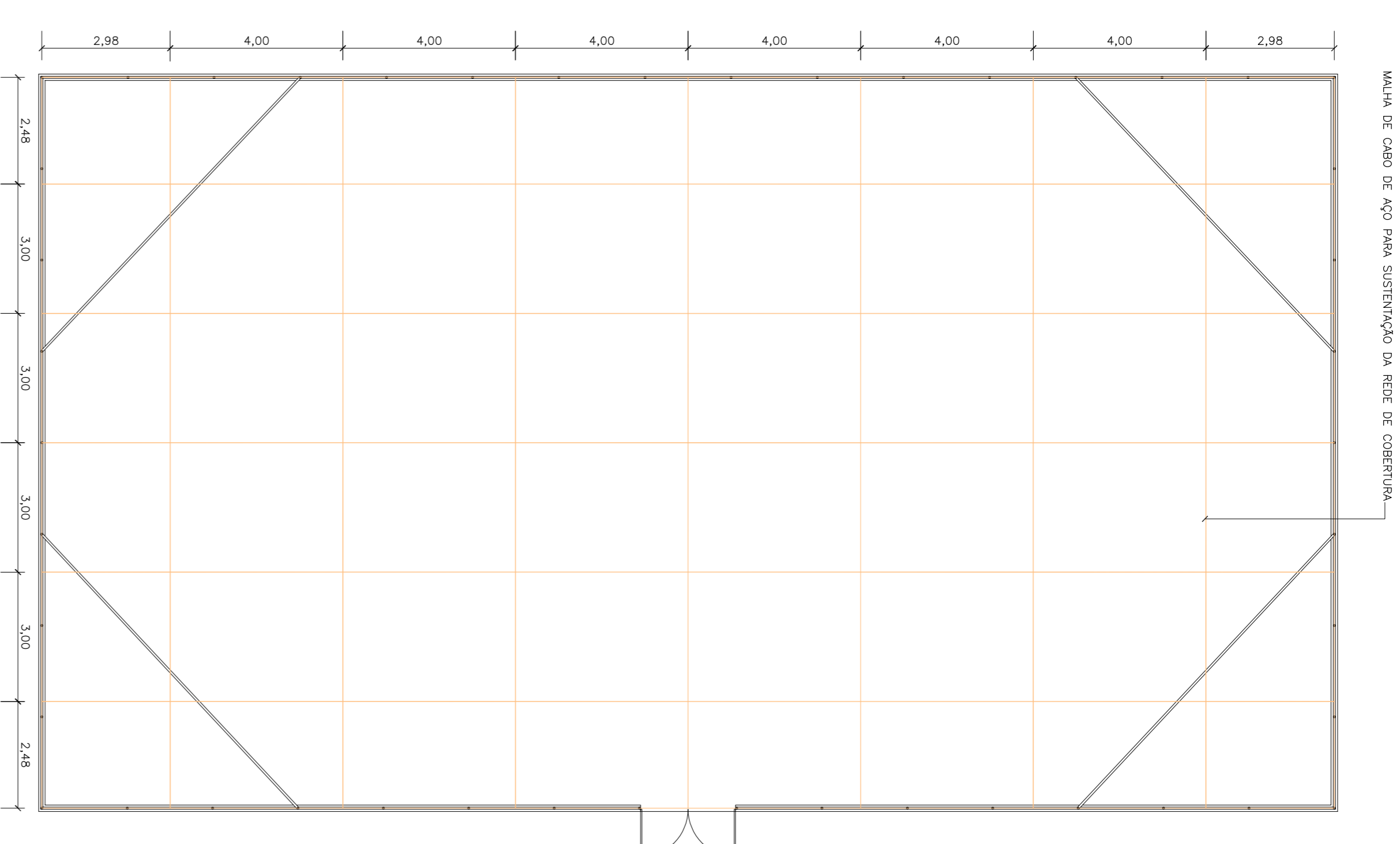
4 COBERTURA - QUADRA ESCALA 1:100
